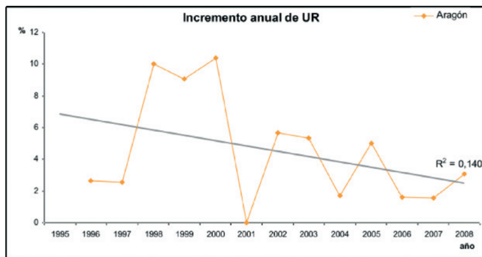
Incremento anual de unidades reproductoras (UR) de la población de quebrantahuesos en Aragón (España) 1995-2008. Se presenta la tendencia lineal con su valor del coeficiente de regresión
